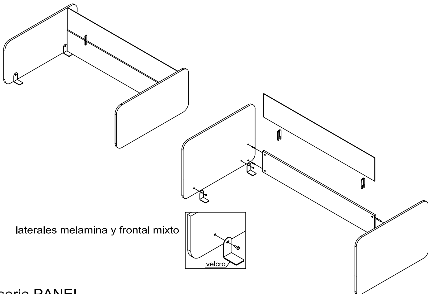
laterales y frontal mixtos
